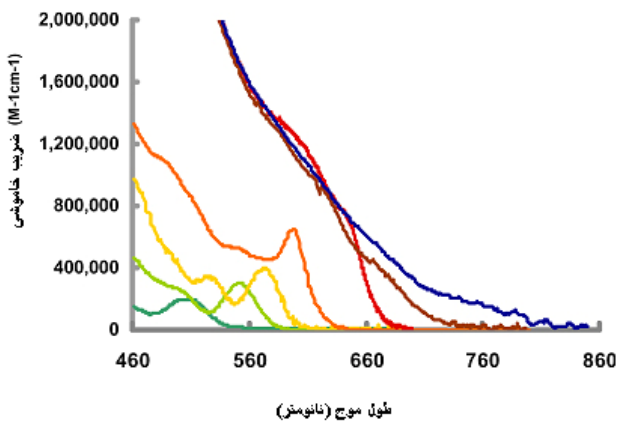
شکل ۲. الف) طیف جذبی و ب) طیف تابشی نقاط کوانتومی مختلف. برگرفته از منبع [۱]
