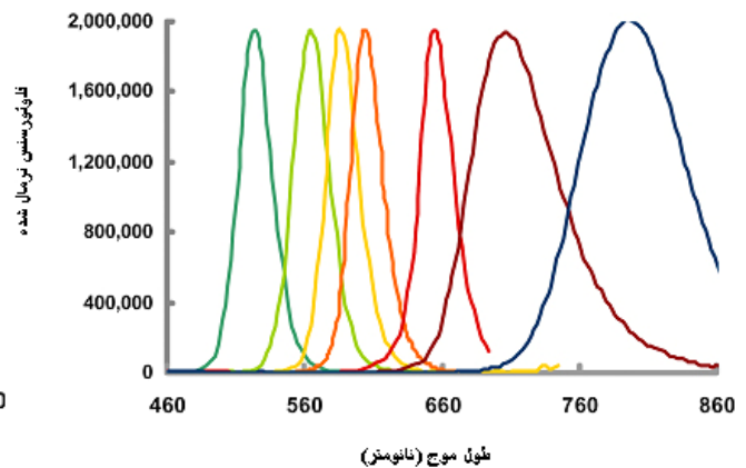
شکل ۲. الف) طیف جذبی و ب) طیف تابشی نقاط کوانتومی مختلف. برگرفته از منبع [۱]
